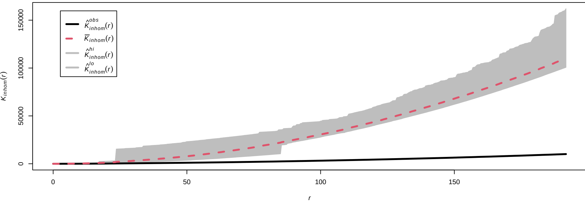
Monte Carlo test för subjekt 14 som är klass 2 mot gruppen 2
