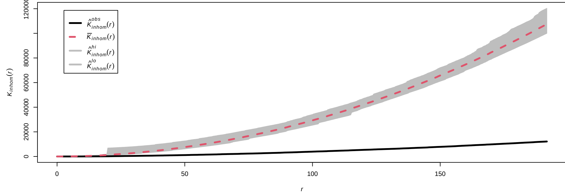
Monte Carlo test för subjekt 20 som är klass 2 mot gruppen 2
