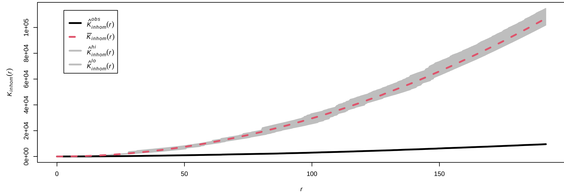
Monte Carlo test för subjekt 4 som är klass 2 mot gruppen 2
