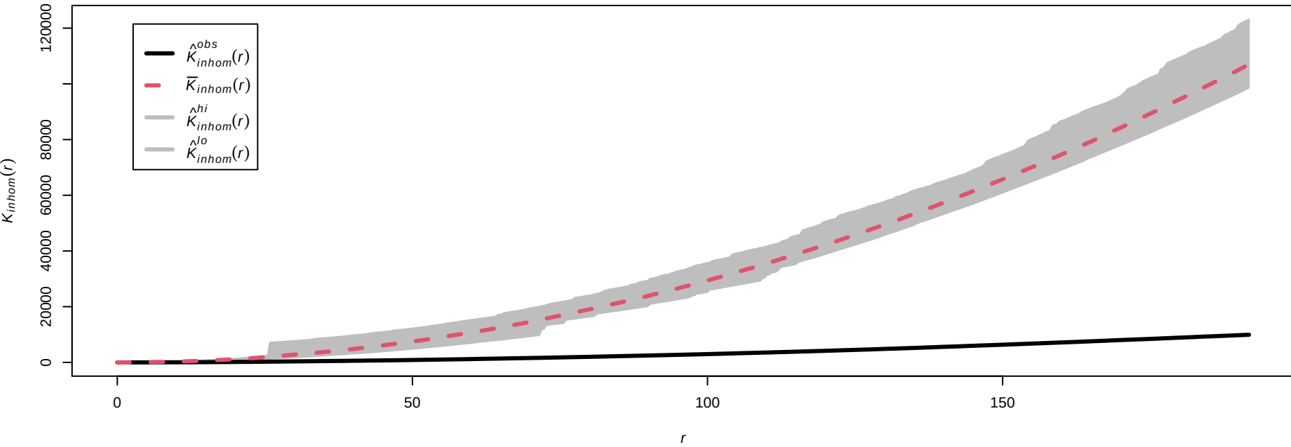
Monte Carlo test för subjekt 19 som är klass 2 mot gruppen 2
