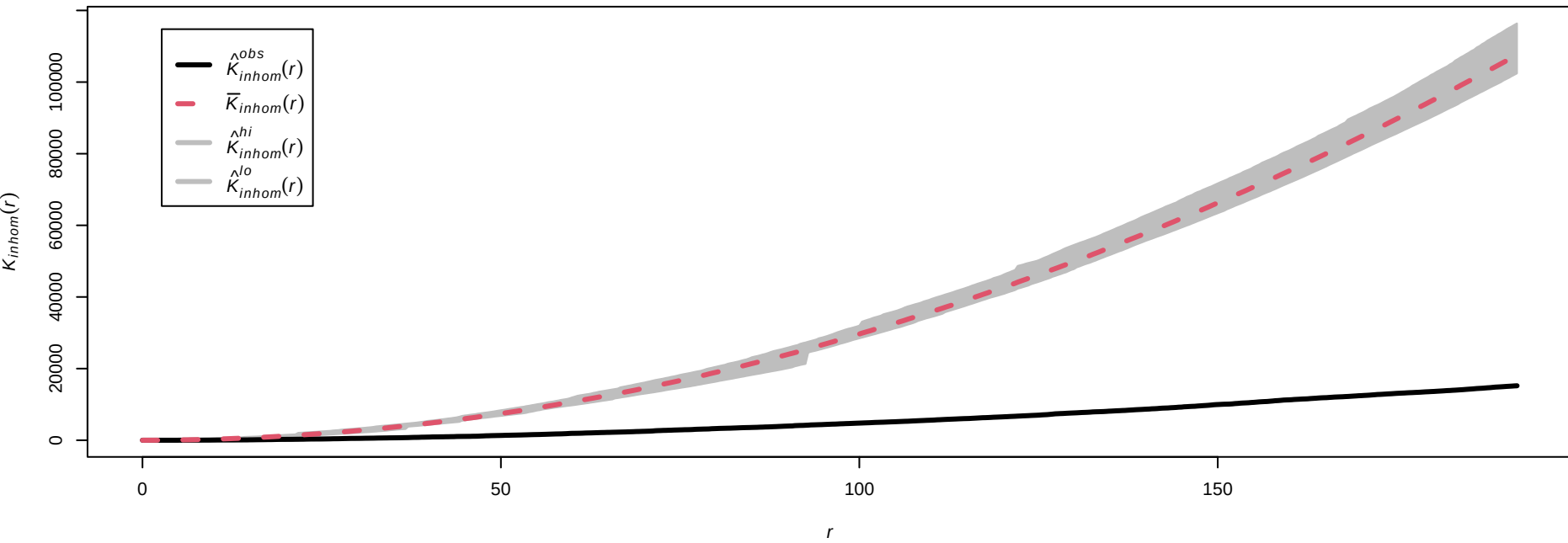
Monte Carlo test för subjekt 7 som är klass 2 mot gruppen 2
