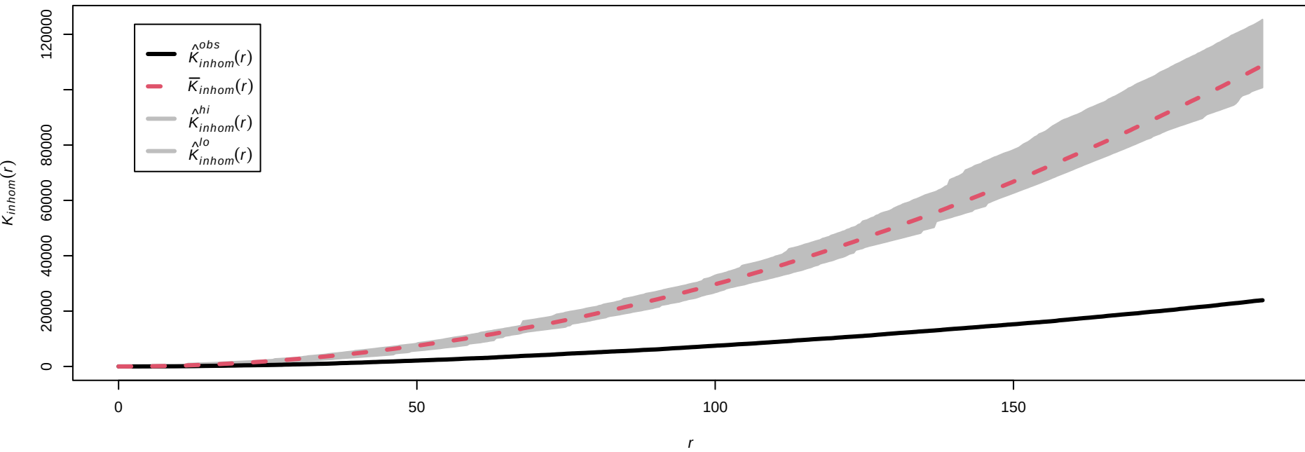
Monte Carlo test för subjekt 3 som är klass 2 mot gruppen 2
