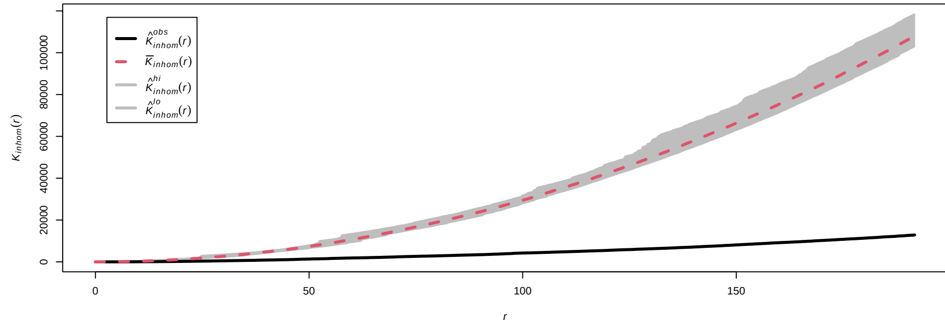
Monte Carlo test för subjekt 15 som är klass 2 mot gruppen 2
