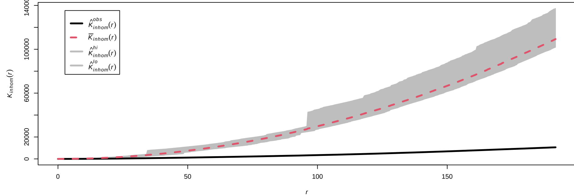
Monte Carlo test för subjekt 8 som är klass 2 mot gruppen 2
